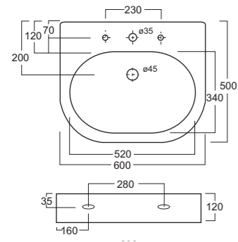
Art. 0852 Lavabo Broadway cm.60 Broadway washbasin cm.60
