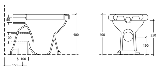
Art. 0158S Vaso a terra scarico pavimento Vaso a terra scarico pavimento
