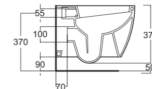
Art. 0650 Vaso Soho sospeso Soho wall hung wc bowl
