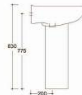
Art. 0857 Lavabo Cleo cm.67 Cleo washbasin cm.67
