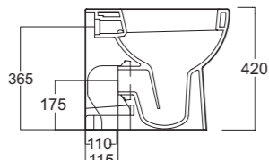
Art. 0150 Vaso Soho Soho wc
