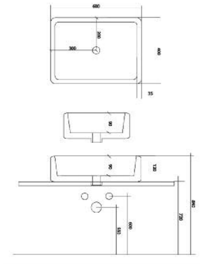
Art. 3132 Lavabo Tendenza senza foro rubinetteria cm. 60 Tendenza washbasin cm.60
