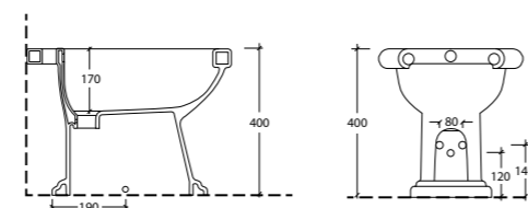
Art. 0558 Bidet 1/3 fori predisposti Bidet 1/3 fori predisposti
